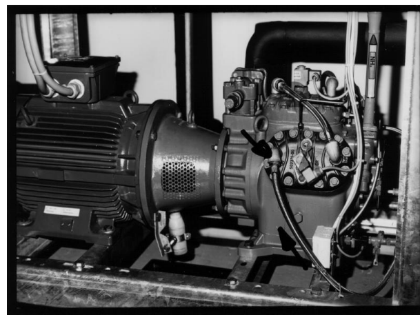
Offener Kältemittelverdichter mit wassergekühlten Zylindern in einer Wasserkühlmaschine für R-717
